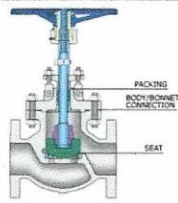
WCB Globe Valves
